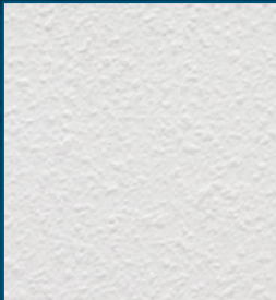
Taburiente
