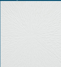
Teneguía
